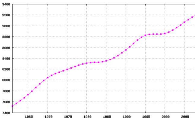
Sveriges befolkningsindex 1960-2010
